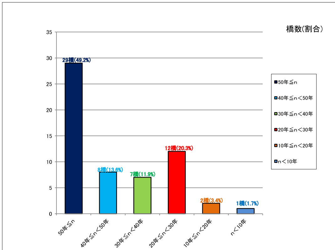
経過年数(n)別の橋数割合
